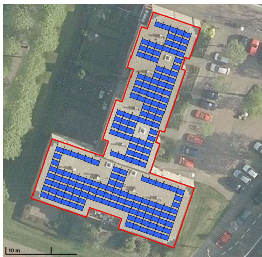
Mogelijke indeling zonnepanelen
