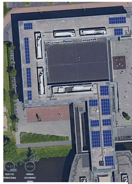
Legplan van de panelen op het dak
